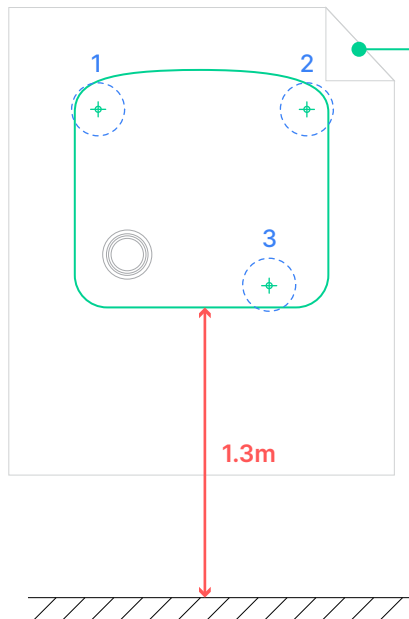
Fig. 4 - Plantilla de perforación para puntos de montaje a estación de carga 1P7K
