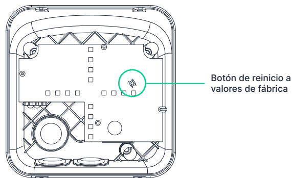
Fig. 15 - Botón de reinicio predeterminado de fábrica (Tradicional)
