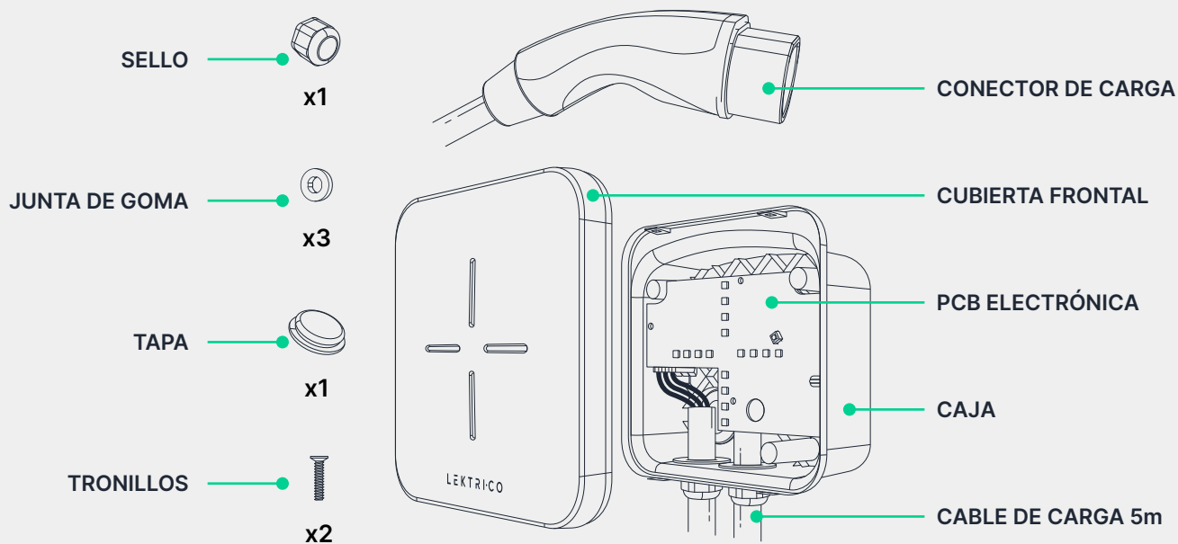
Fig. 1 - Los componentes principales de la estación de carga 1P7K
