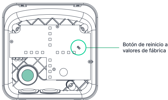
Fig. 14 - Botón de reinicio a valores de fábrica (Nuevo)
