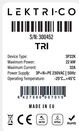
Fig. 2 - Etichetta di prodotto della stazione di ricarica
