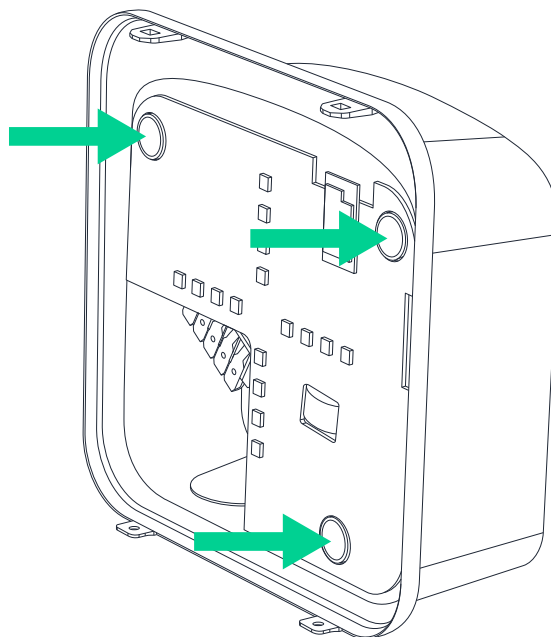
Fig. 6 - Punctele de montare a stației de încărcare
