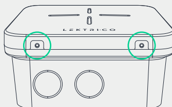
Fig. 11 - Șuruburi de fixare a capacului frontal în partea de jos
