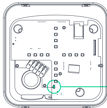
Fig. 14 - Comutator de resetare la valorile implicite din fabrică
