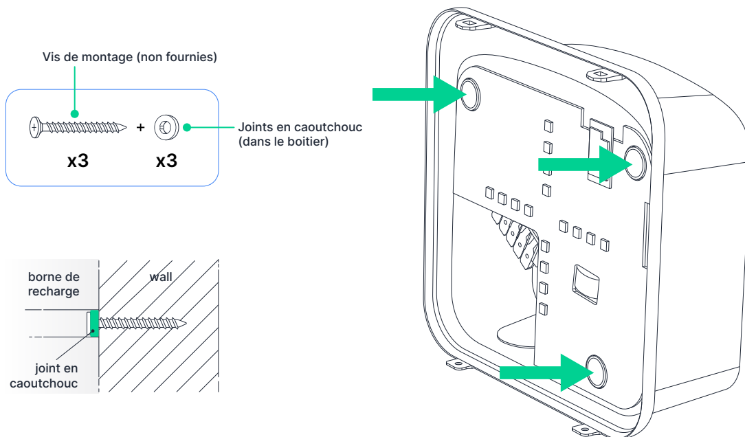
Fig. 6 - Les points de fixation de la borne de recharge
