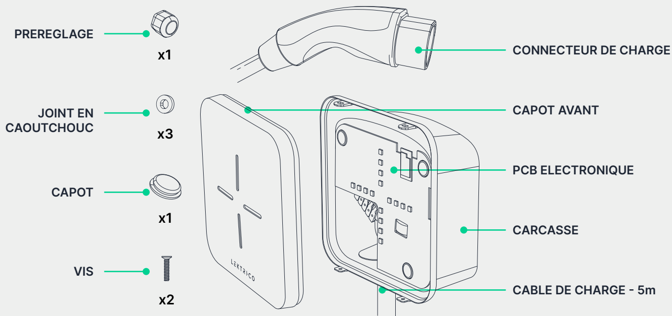
Fig. 1 - Composantes principales de la borne de recharge ONE™
