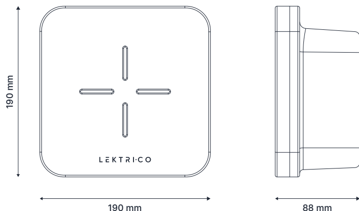
Fig. 12 - Dimensions totales de la borne de recharge
