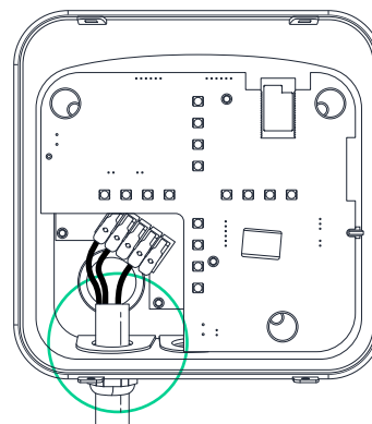
ZONE DE DÉCOUPE EN BAS À GAUCHE
