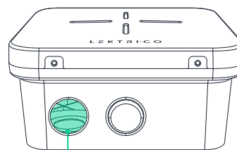
ZONE DE DÉCOUPE EN BAS À GAUCHE
