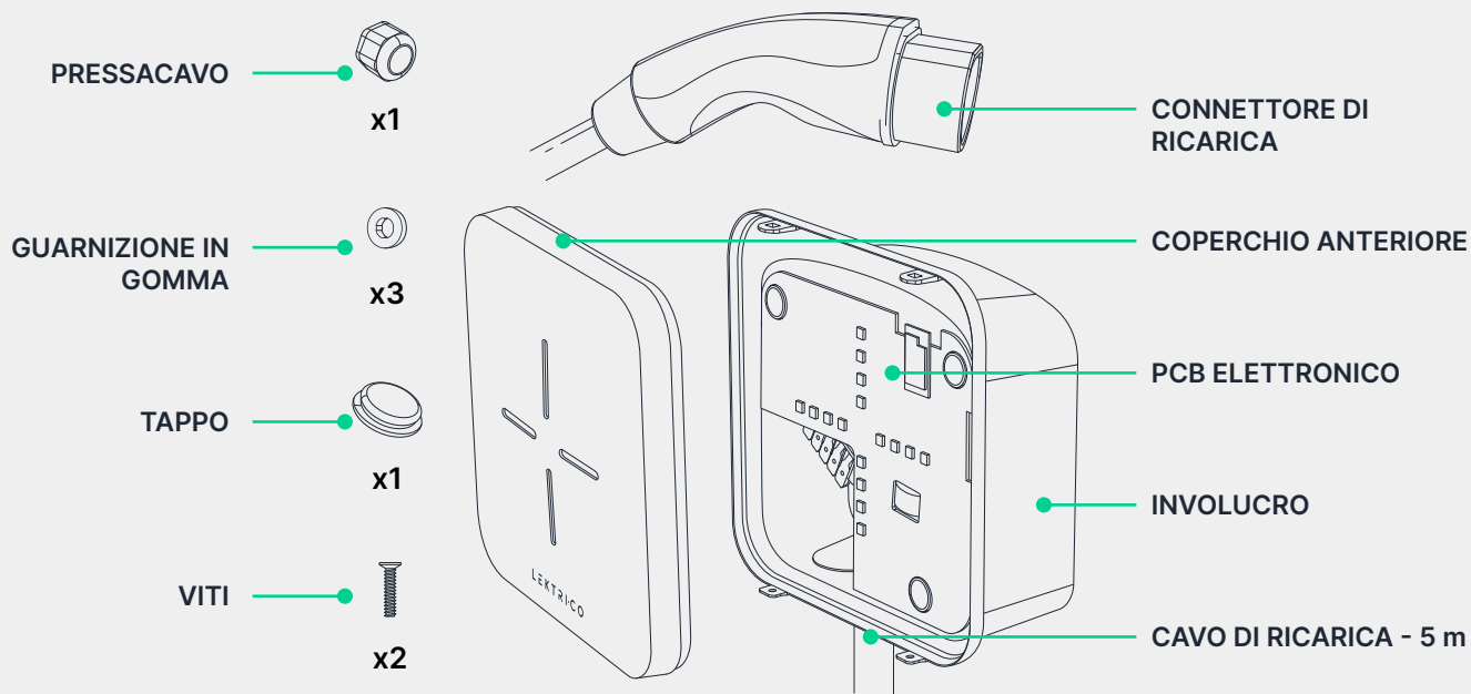
Fig. 1 - Componenti principali della stazione di ricarica ONE™
